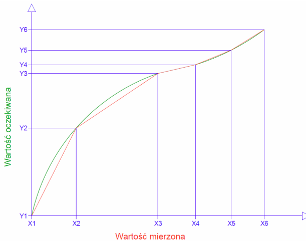
Rys. 11: Przykład charakterystyki indywidualnej.
