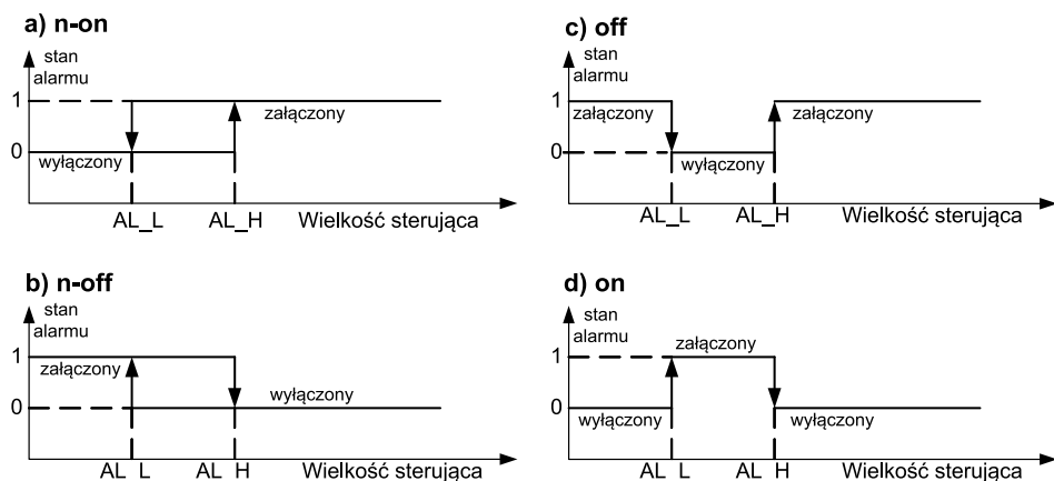
Rys. 12: Typy alarmów: a) n-on; b) n-off; c) off; f) on.
