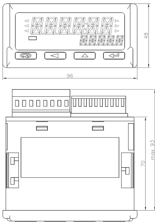
Rys. 3: Gabaryty miernika.
