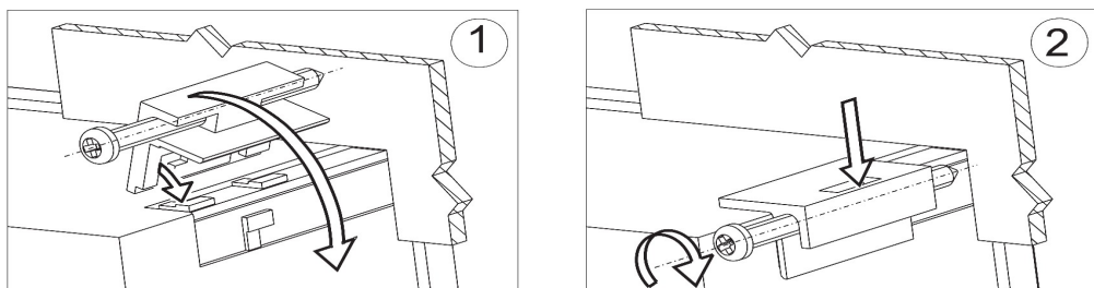
Rys. 2: Mocowanie miernika.
