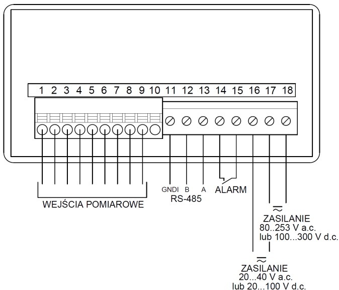
Rys. 5: Sygnały na listwach zaciskowych.
